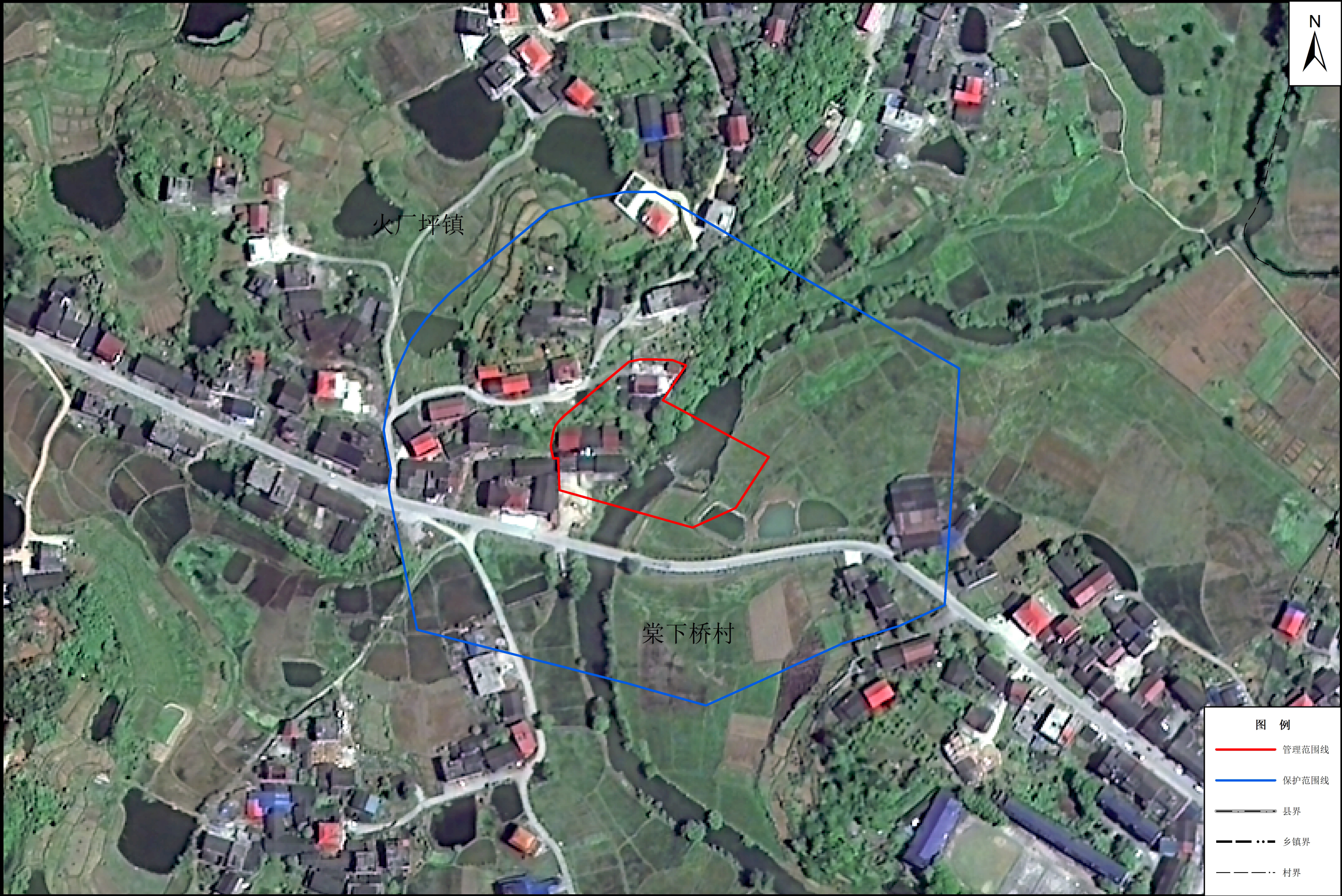
棠下桥坝水闸管理与保护范围划界成果示意图
